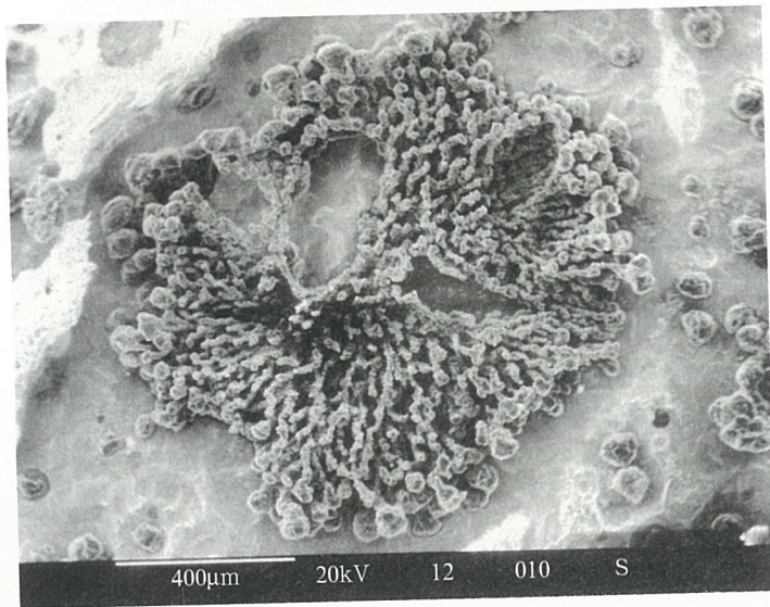
图 3-69 碎块状石墨共晶团的结构 a) 热碱液蚀显 b) 三维结构 (SEM 观察) [1]
