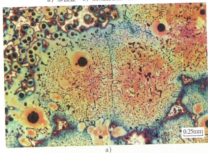
图 3-68 灰斑区的碎块状石墨共晶团组织 a) 未蚀显 b) 热碱液蚀显 (同一视场)
