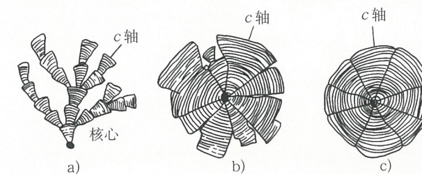
图 3-71 碎块状石墨的生长模型 [113]
