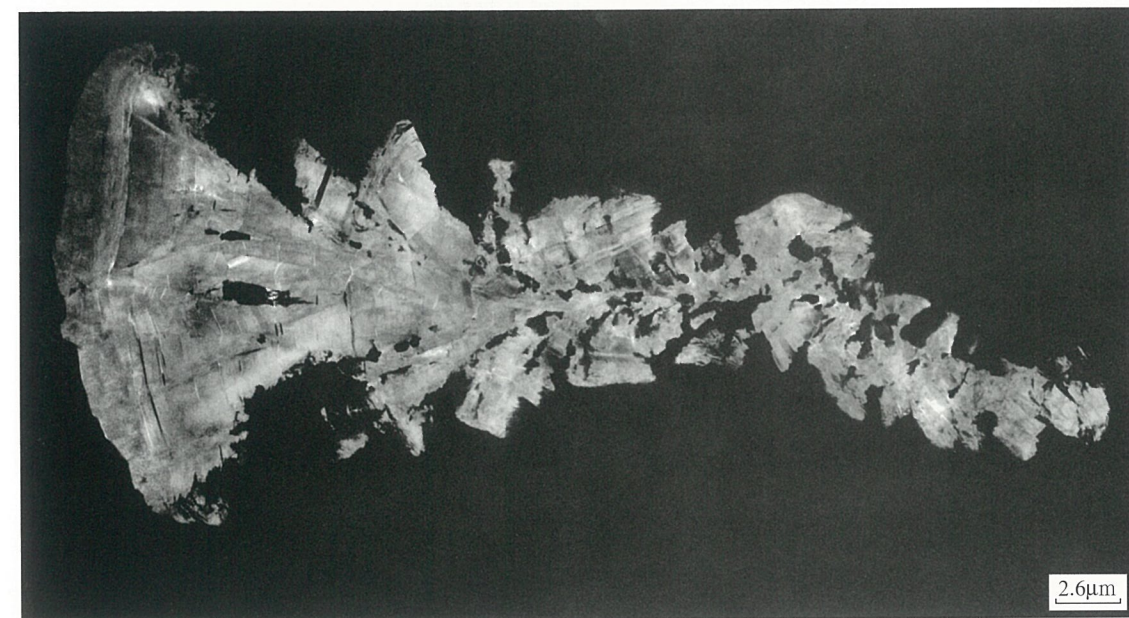
图 3-70 碎块石墨分枝的结构 [1]
