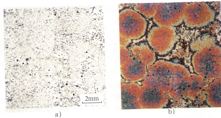
图 3-68 灰斑区的碎块状石墨共晶团组织 a) 未蚀显 b) 热碱液蚀显 (同一视场)
